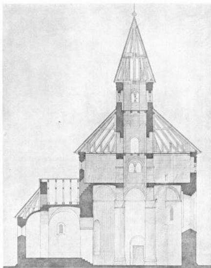
Tværsnit af kirken, set fra nord Fra Danmarks Kirker
